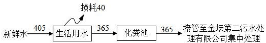
图 2-1 项目实际水平衡图（t/a）
