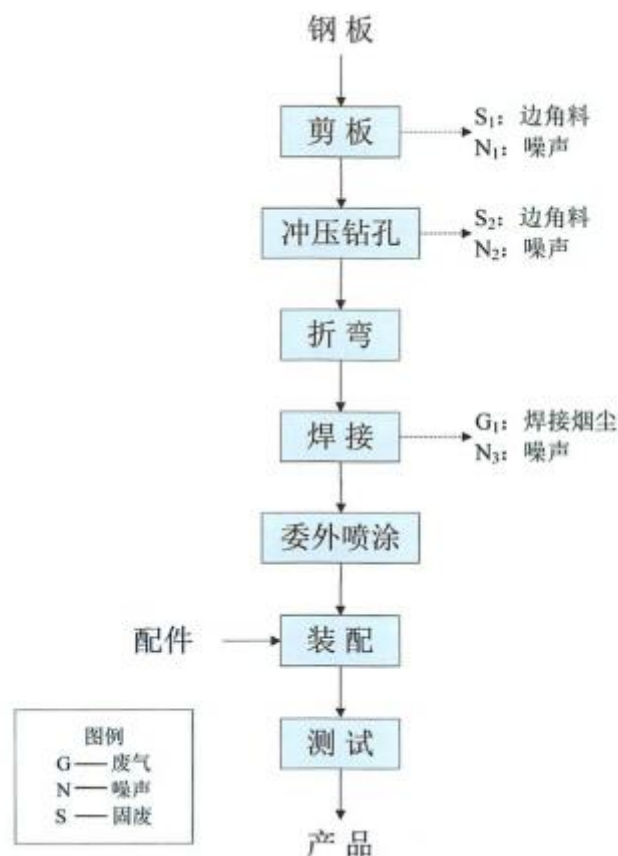
图 2-2 教学实验仪器生产工艺流程图
